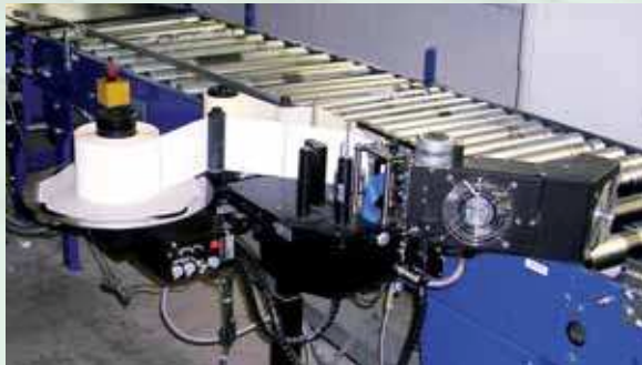
Etichettatore per l'applicazione automatica di una etichetta "ad angolo" sul fronte e lato del collo. Labelling system for applying a label on the front and on the side of the parcel.
